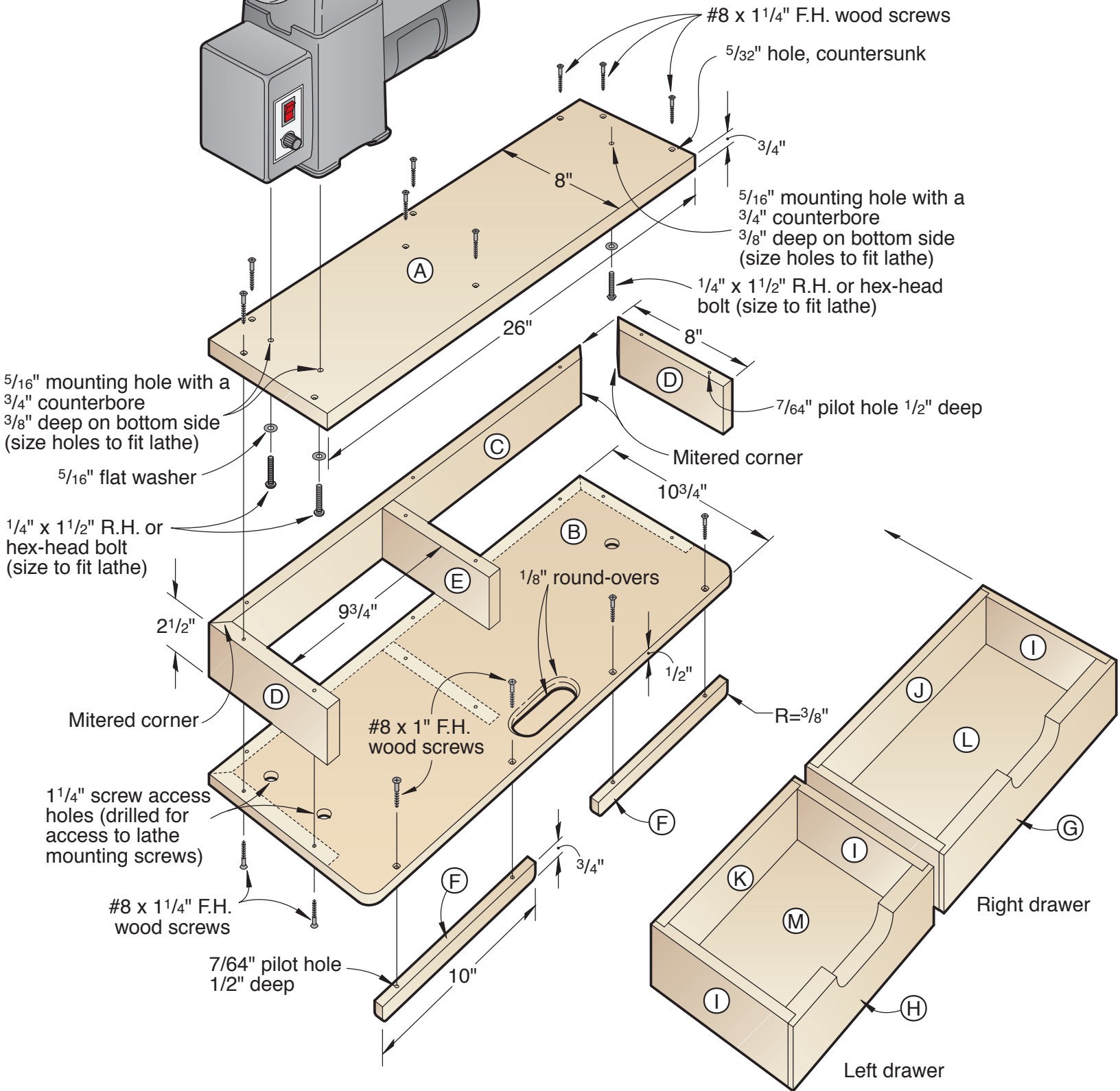
Mini lathe
